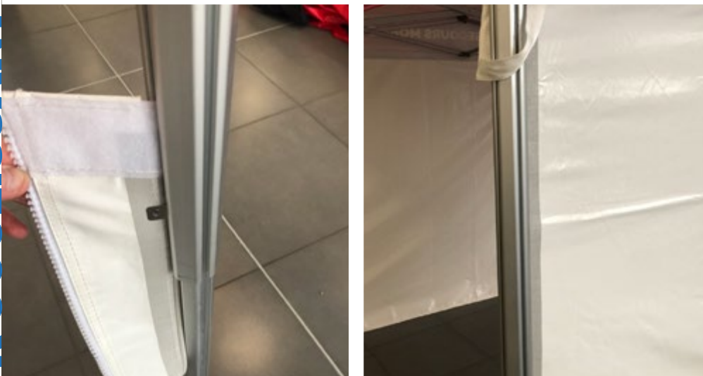
Système de mur à jonc coulissant directement dans le profilé
